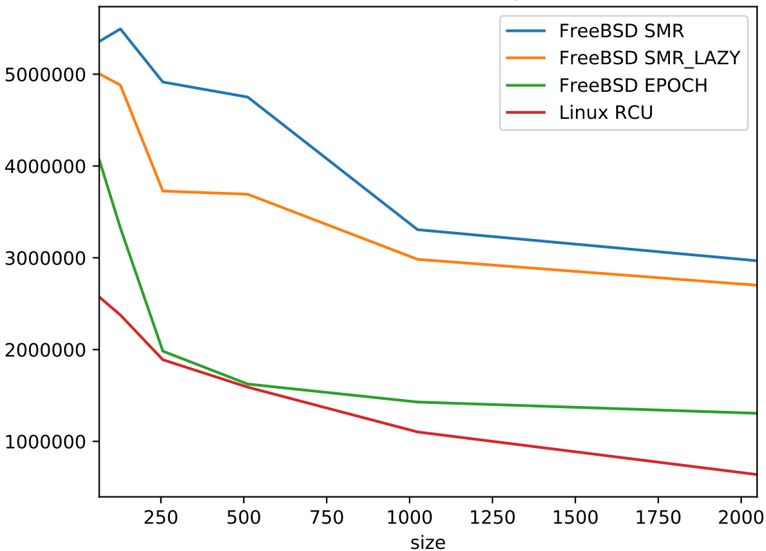
FreeBSD vs Linux ops/s
